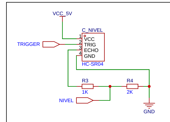
SENSOR DE CONTROL DE NIVEL HC-SR04
