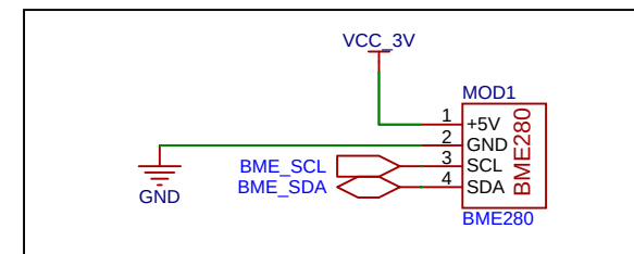
SENSOR DE PRESION, TEMPERATURA Y HUMEDAD
