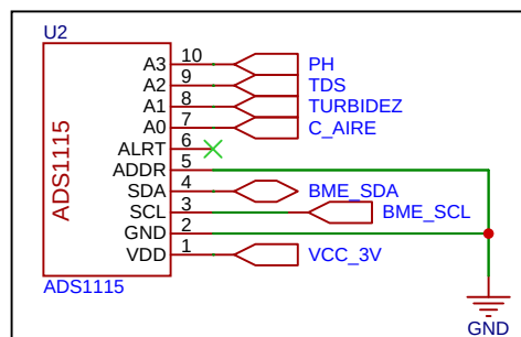
CONVERTIDOR ANALOGICO DIGITAL ADS1115
