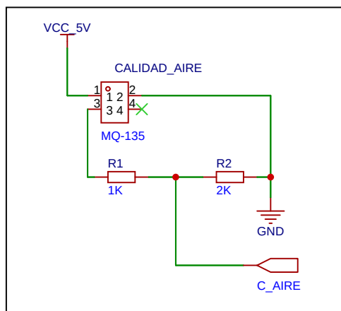
SENSOR DE CALIDAD DEL AIRE MQ-135
